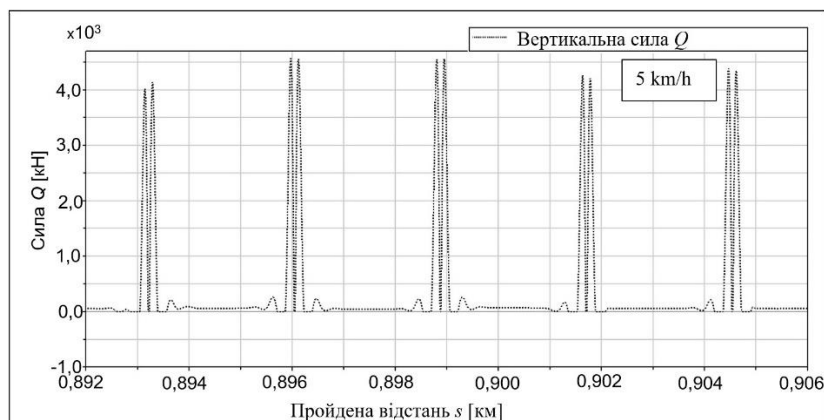
Рисунок 3 – Значення сили Q , що діє на пошкоджене колеса при швидкості руху 5 км/год
