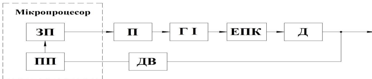
Рисунок 1 – Функціональна схема системи автоматичного регулюванні витрати абразивного матеріалу
