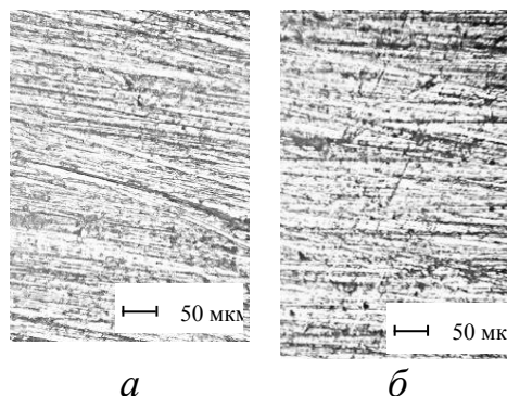
Рисунок 2 – Морфологія поверхонь тертя при зношуванні о закріплені частинки абразиву наплавленого сплаву ПГ-10Н-01 (а) і КМ (20% МКМ + 80% ПГ-10Н-01) (б)
