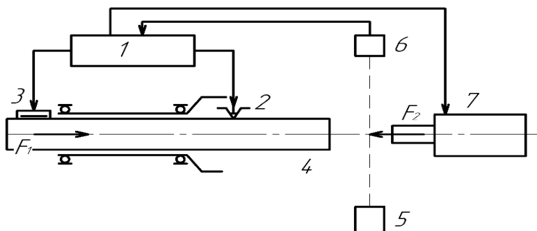
Рисунок 1 – Структура системи виставлення торця заготовки
