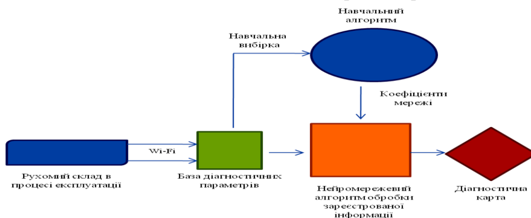
Рисунок 1 – Алгоритм оцінки технічного стану рухомого складу за допомогою нейромережевого моделювання
