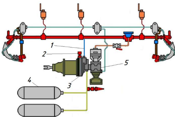
Рисунок 1 – Модернізована пневматична схема пасажирського вагона
