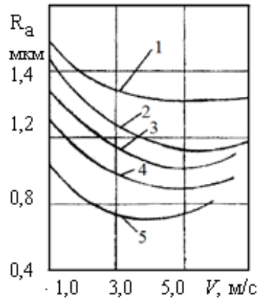
Рисунок 2 – Вплив структури чавуну на висоту мікронерівностей поверхні після обробки мінералокерамікою BOK71
