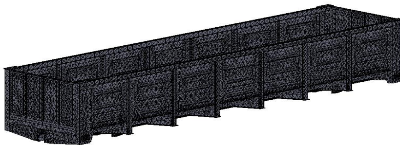
Рисунок 1 – Скінчено-елементна модель несучої конструкції кузова напіввагона
