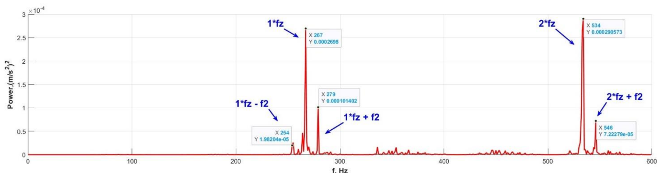
Рисунок 2 — Спектр потужності вібрації ТЗП після процедури ДМЕ
