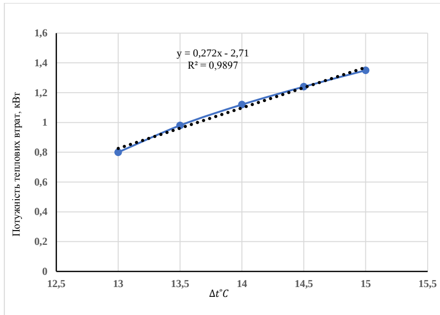
Рисунок 1 – Потужність теплових втрат салону від \Delta t °C
