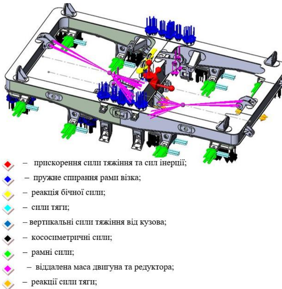
Рисунок 2 – Приклад розрахункової моделі рами візка ДС3 (режим Па)
