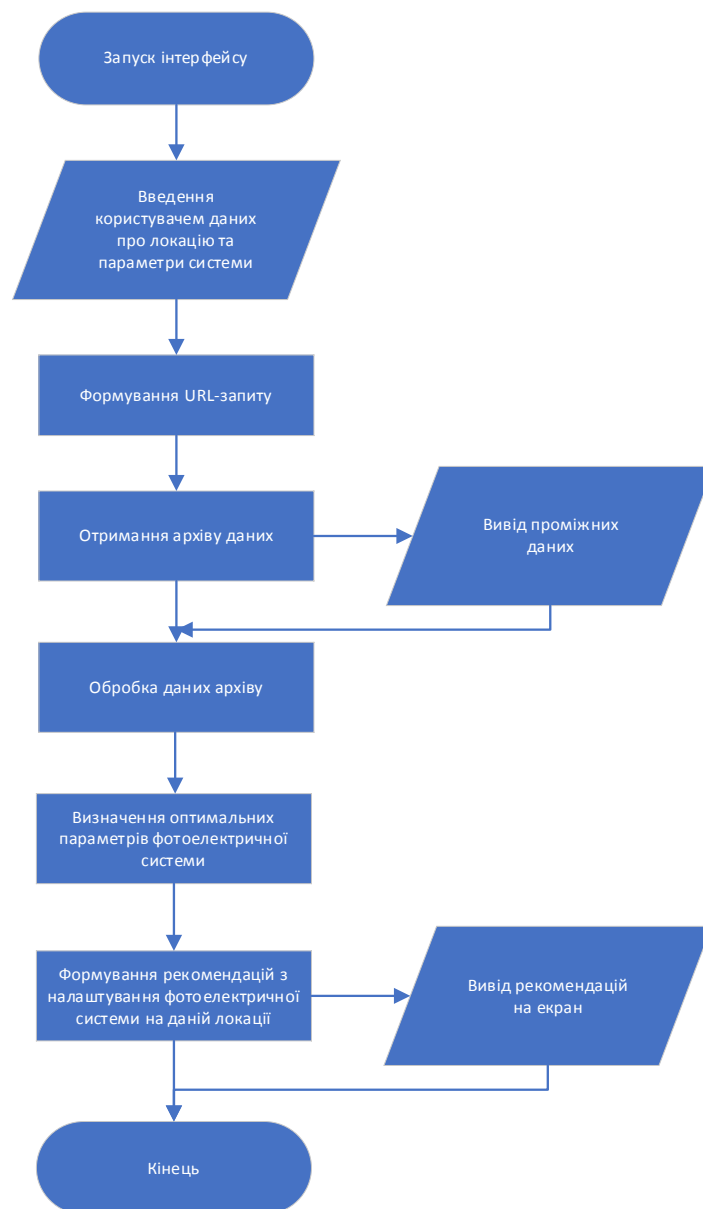
Рисунок 1 – Функціональна блок-схема програми
