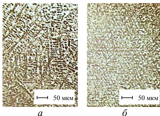
Рисунок 1 – Мікроструктура наплавлених покриттів: а – ПГ-10Н-01; б – КМ (20% МКМ + 80% ПГ-10Н-01)
