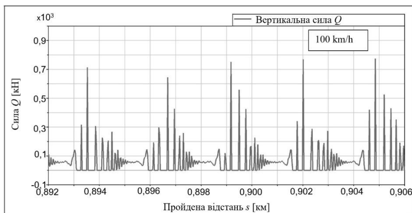
Рисунок 4 – Значення сили Q , що діє на пошкоджене колесо при швидкості руху 100 км/год
