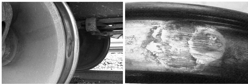
Рисунок 1 – Повзун на поверхні кочення залізничного колеса
