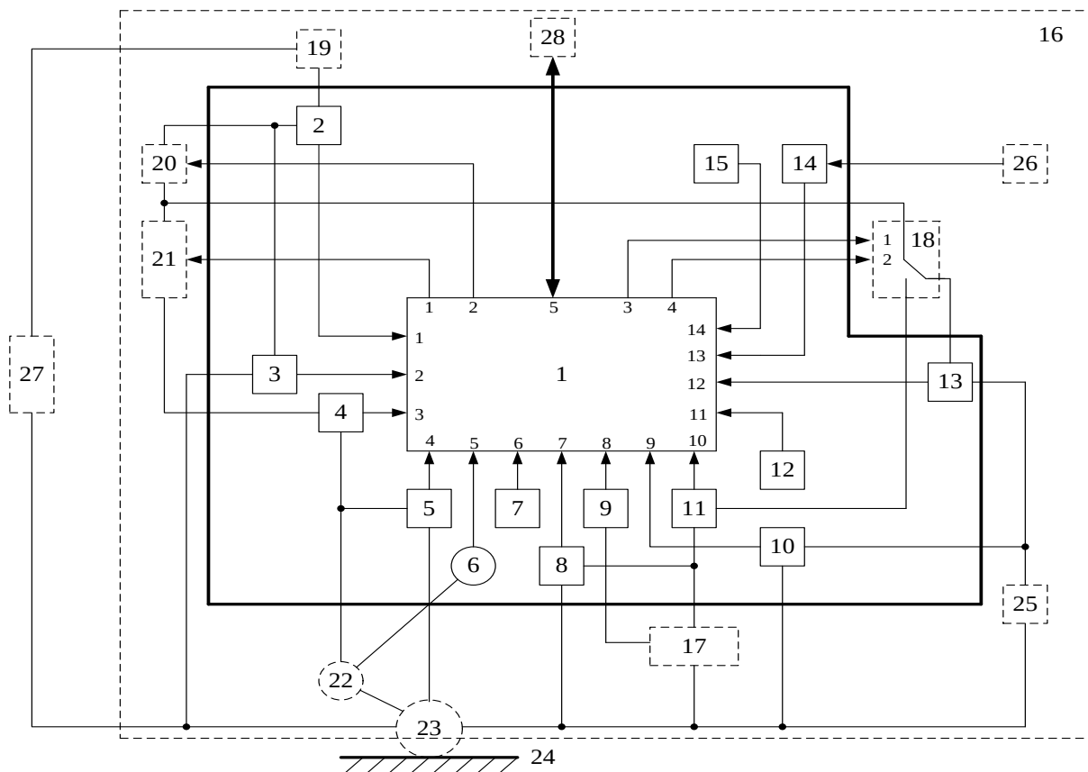
Рисунок 1 – Блок-схема системи керування енергообмінними процесами
