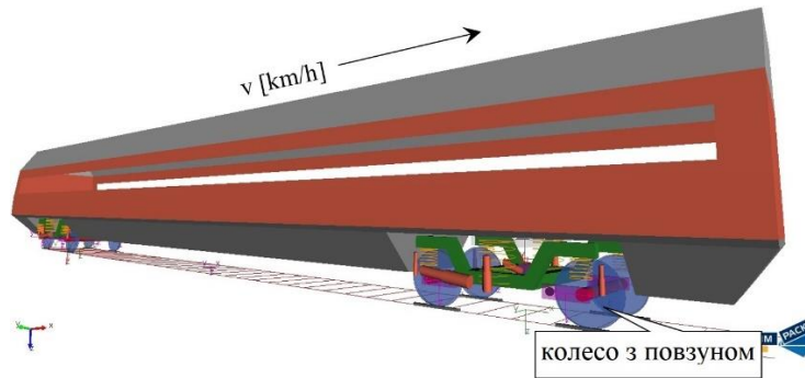
Рисунок 2 – Модель рейкового транспортного засобу з пошкодженим колесом
