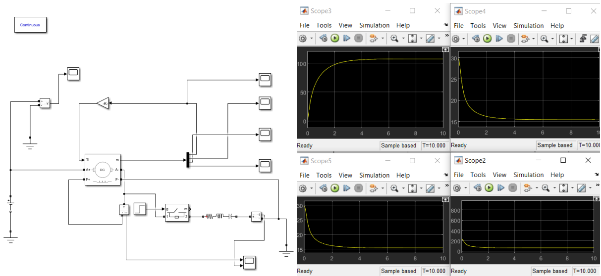
Рисунок 3 – Модель та осцилограми отримані в результаті розрахунку тягового електричного двигуна постійного струму з послідовним збудженням з заданими параметрами побудованого в середі MATLAB SIMULINK R2022b
