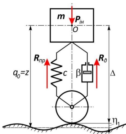
Рисунок 1 – Розрахункова схема коливальної системи з гідравлічним гасником коливань, що реалізує сили в'язкого тертя: c – жорсткість пружного зв'язку; \beta – коефіцієнт дисипації гасника; \eta – амплітуда нерівності; m – маса, що припадає на одне колесо; z – абсолютне переміщення; \Delta – відносне переміщення (прогин)
