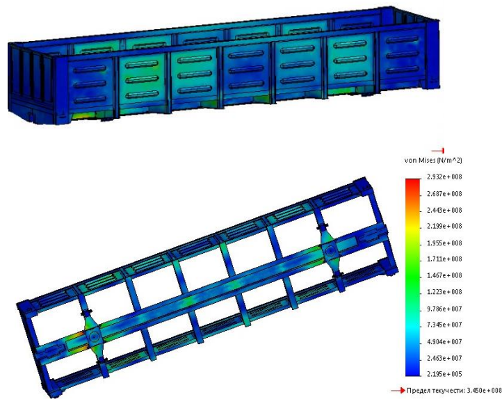
Рисунок 2 – Приклад епюри навантаження напіввагона
