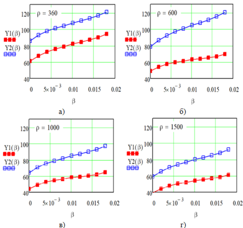
Рисунок 1 – Розрахункові залежності спрямовуючого гребневого зусилля Y(\beta) (кН) від кутів перекосу колісних пар \beta (рад), швидкості руху і радіусу кривої: Y1(\beta) – швидкість руху 20 м/с (72 км/год); Y2(\beta) – 27 м/с (100 км/год); а) для радіусу кривої \rho = 360 м; б) \rho = 600 м; в) \rho = 1000 м; г) \rho = 1500 м
