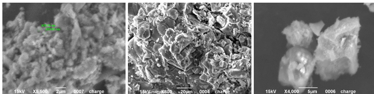
Рисунок 1 – Нано- та дисперсні алмази у конгломератах детонаційної шихти
