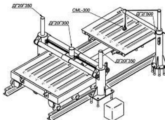
Рисунок 4 – Установка правки люків напіввагонів
