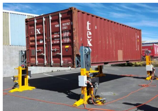
Рисунок 1 – Робота C-Lift A32
