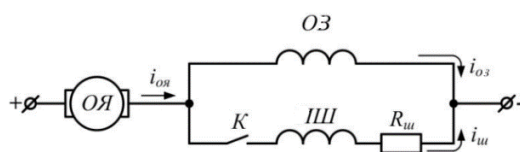
Рисунок 2 – Шунтування обмотки збудження резистором
