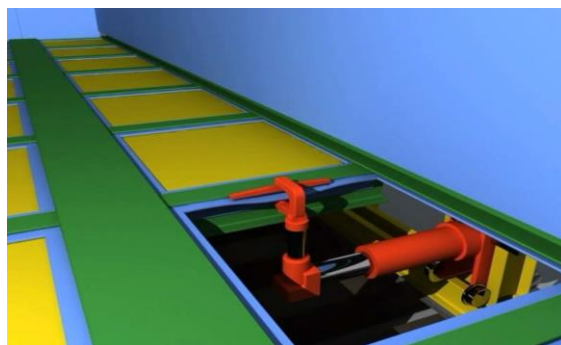
Рисунок 2 – Механізм для виправлення рамок люків універсальної ВРМ
