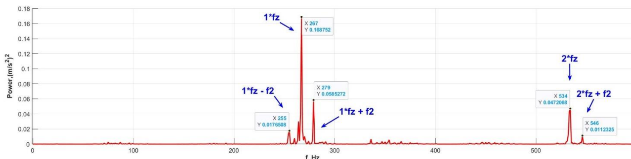
Рисунок 1 – Спектр потужності вібрації ТЗП електропоїзда EP2
