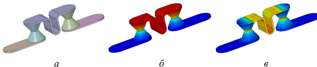
Рисунок 1 – Термоелектричний елемент з напівпровідниками в формі усічених конусів та компенсованою комутаційною пластиною: а – геометрична модель; б, в – відповідно розподіл температури t [ ^{\circ}\text{C} ] в діапазоні [0; 3,1] та густини теплового потоку q [ \text{Wt/m}^2 ] в діапазоні [0; 332,2] при силі робочого струму I=0,1 А (синій, блакитний кольори – мінімальні значення діапазону; зелений, жовтий кольори – середні значення діапазону; рудий, червоний кольори – максимальні значення діапазону)
