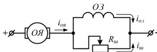
Рисунок 1 – Двигун з послідовним збудженням, облаштований шунтуванням обмотки збудження резистором
