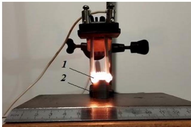
Рисунок 1 – Ініціювання СВС-процесу (1 – ніхромові спіраль; 2 – зразок з шихти)
