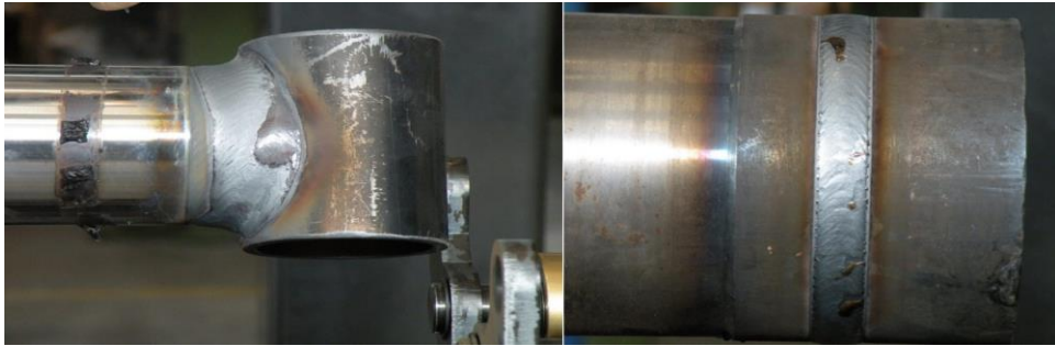
Рисунок. 1 – Приклад шва, отриманого з допомогою зварювальної установки Joda Horizontal виробництва Carpano Equipment [1]
