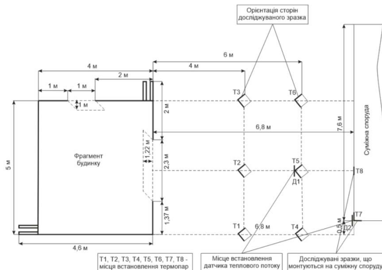
Рис. 4. Схема улаштування випробувальних зразків та вимірювальної техніки
