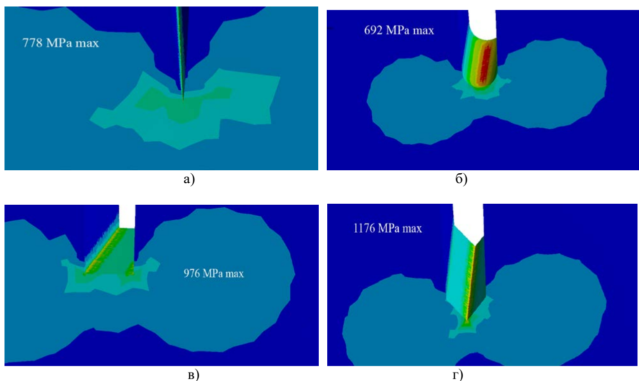
Рис. 1. Напружено-деформований стан брусу з різними засобами моделювання вістря тріщини: а – тріщина у вигляді призми; б – вістря тріщини у вигляді напівциліндра; в – тріщина у вигляді паралелепіпеда; г – вістря тріщини у вигляді призми.
