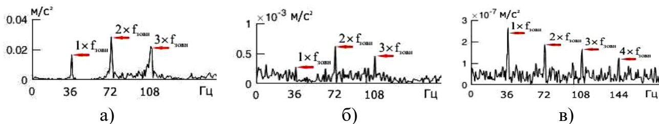
Рис. 1. Спектри обвідної вібрації буксового підшипника кочення: а — за результатом моделювання; б — за результатом експериментальних досліджень; в — спектр квадратичної обвідної вібрації за результатом експериментальних досліджень
