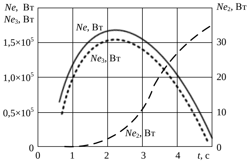
Рис. 1. Визначення реалізованої потужності двигуна при русі на повороті
