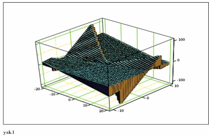
Рис. 2. Залежність коефіцієнта перетворення y_{sk+1} відліку u_k напруги вхідного сигналу від його величини при фіксованих величинах u_{k+1}
