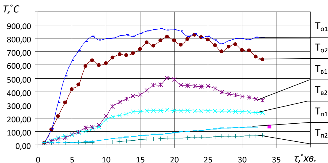
Рис. 2. Середня температура у 3-х зонах кабельного тунелю: T_{o1} – у верхній частині тунелю зони осередку пожежі; T_{o2} – у нижній частині тунелю зони осередку пожежі; T_{b1} – у верхній частині тунелю зони між осередком пожежі та отвором для виходу продуктів горіння; T_{b2} – у нижній частині тунелю зони між осередком пожежі та отвором для виходу продуктів горіння; T_{n1} – у верхній частині тунелю зони між осередком пожежі та місцем підпору повітря; T_{n2} – у нижній частині тунелю зони між осередком пожежі та місцем підпору повітря.
