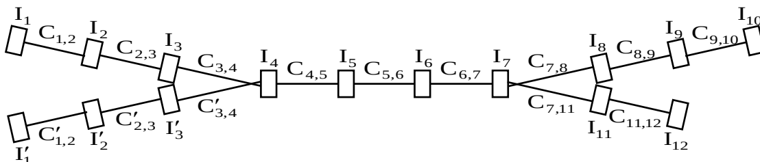
Рис. 1. Вихідна 15-масова еквівалентна динамічна схема ШПУ
